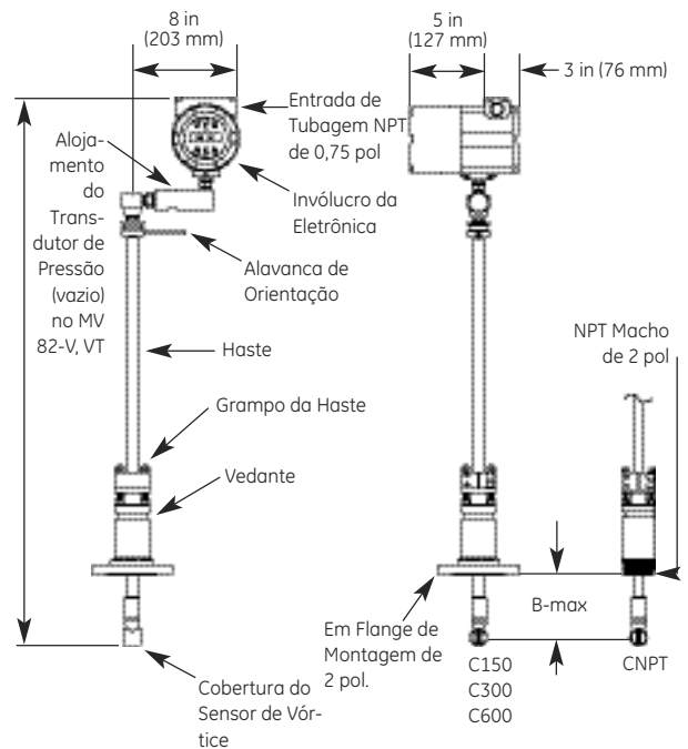
Esquema Dimensional: Modelos de Material de Encapsulamento
